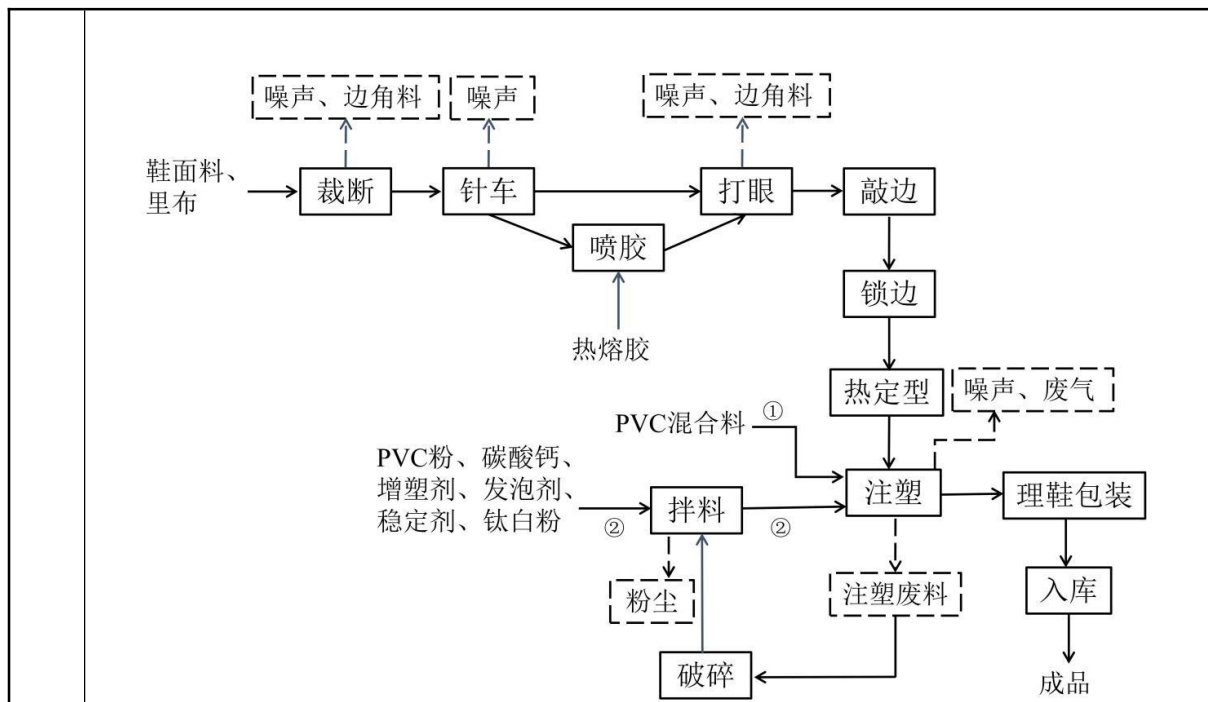
图 2-1 注塑鞋生产工艺流程及产污环节示意图
